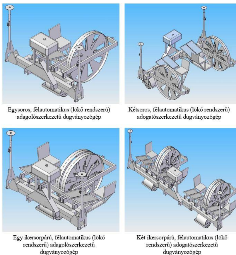
3. ábra. Félautomatikus adogatószerkezetű dugványozógépek elvi kialakítása (forrás: Horváth - Vágvolgyi, 2021a)
