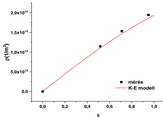
1. ábra. Hengerelt lemezek keménysége alapján számolt diszlokációsűrűség a deformáció függvényében
