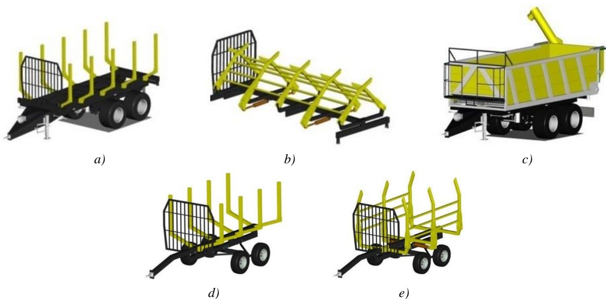
4. ábra. Az erdészeti többcélú kihordó különböző gépcs család gépei: a) merev rakoncás felépítményű kihordó; b) mozgó rakoncás felépítmény; c) aprító-szállító kihordó; d) merev rakoncás felépítményű könnyű kihordó; e) mozgó rakoncás felépítményű könnyű kihordó (forrás: Horváth B.)
