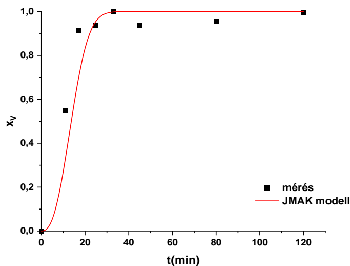
2. ábra. Lemezek újrakristályosodott térfogataránya a hőkezelési idő függvényében 450°C-on
